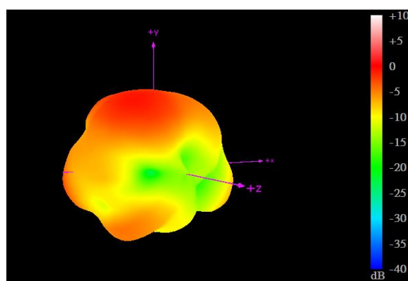
960MHz
