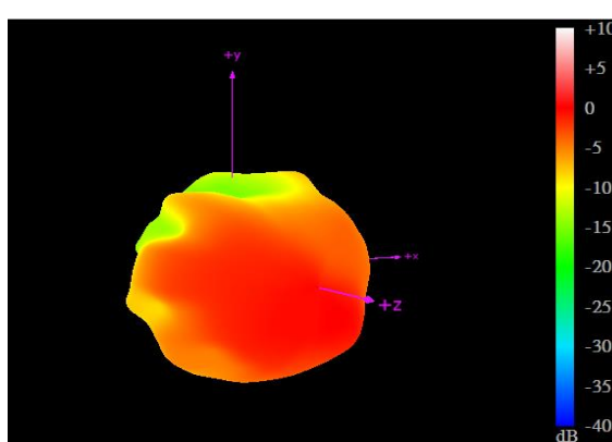
2170MHz
