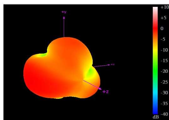
960MHz
