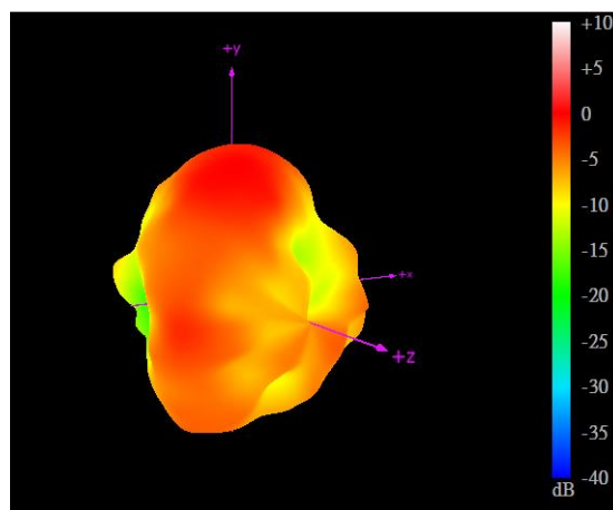
3500MHz
