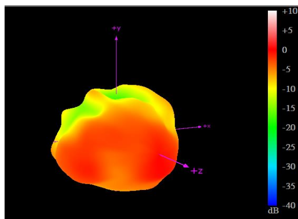
2170MHz
