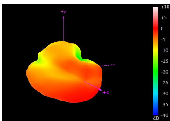
2170MHz
