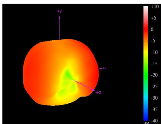
704MHz
