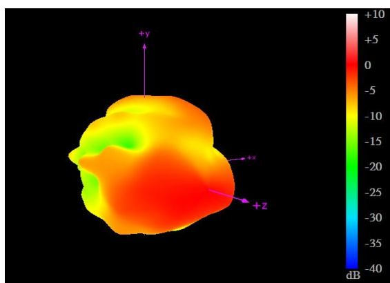
2690MHz
