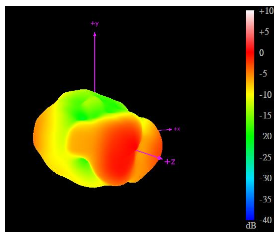
2170MHz
