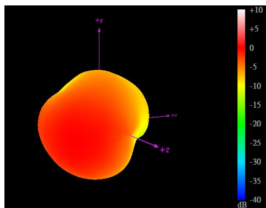
704MHz
