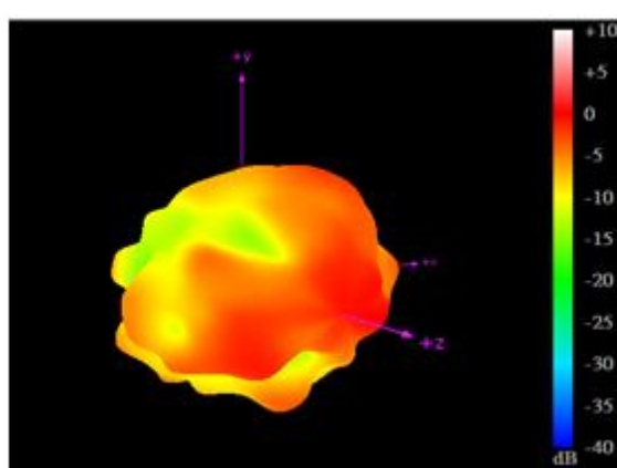
3500MHz
