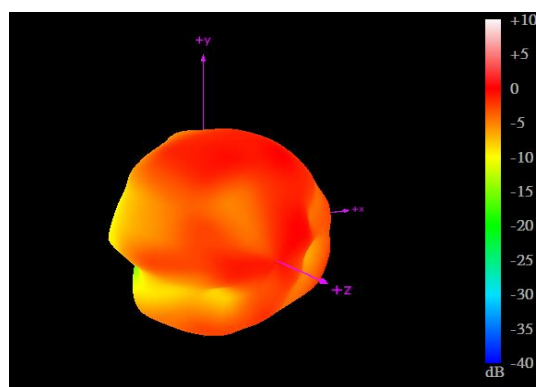
3500MHz
