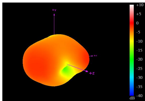
704MHz
