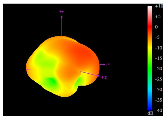
960MHz
