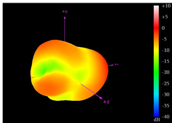
704MHz
