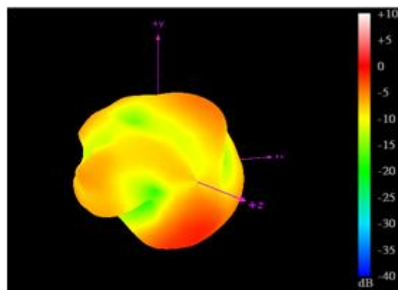
960MHz
