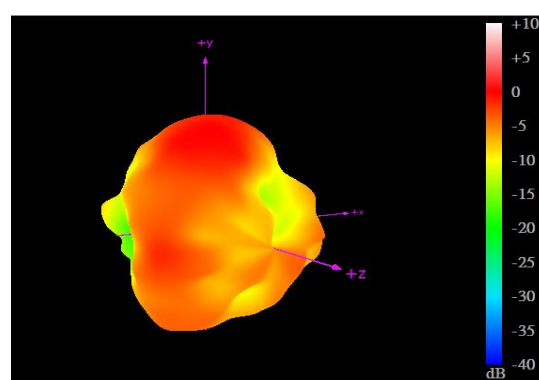
3500MHz
