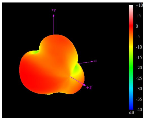
960MHz
