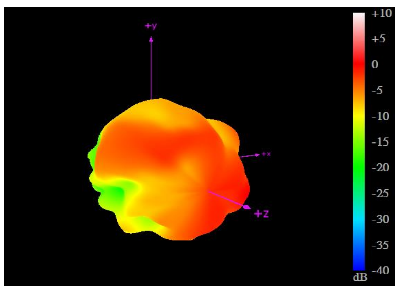
5550MHz
