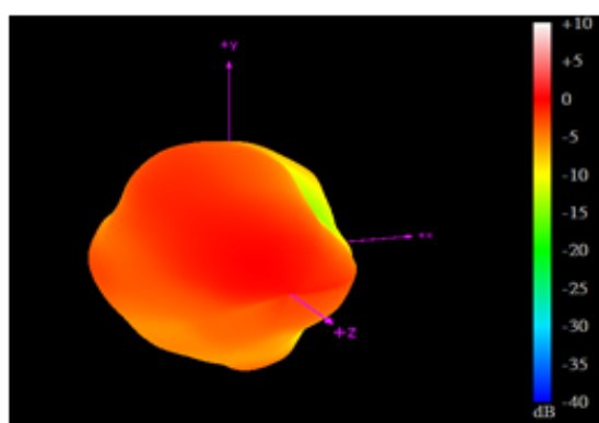
1710MHz
