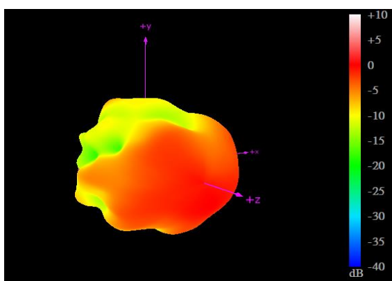
1710MHz
