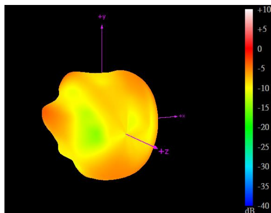
960MHz
